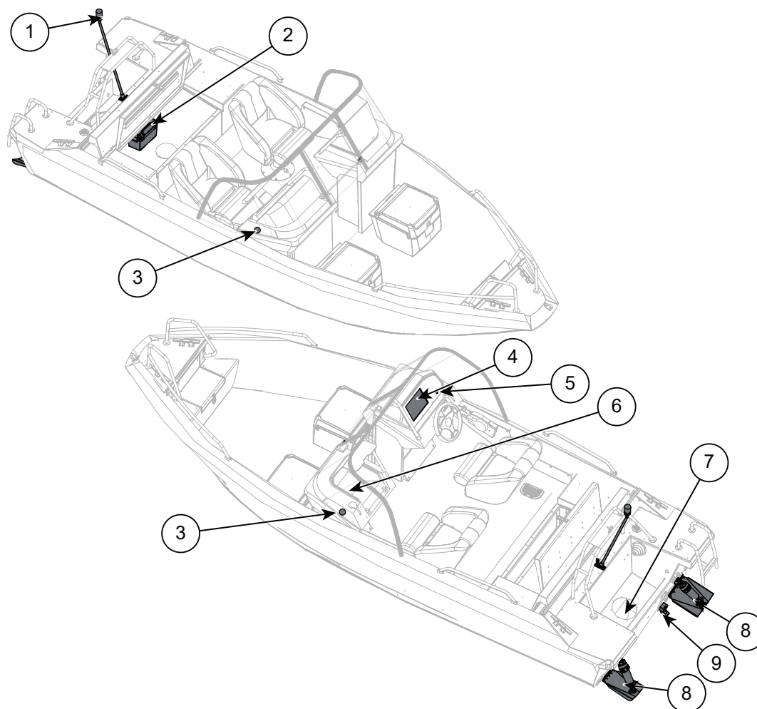
Figur 8.2 Buster X elektrisk utrustning
