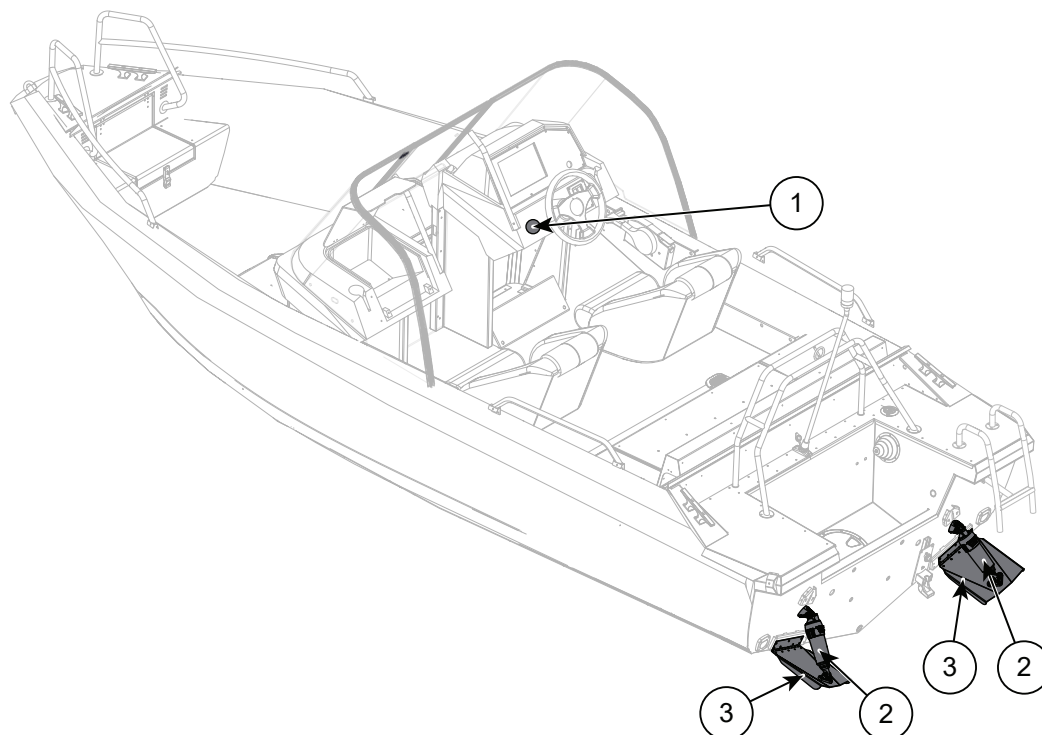
Figur 5.4 Komponenter till Buster X trimsystem
