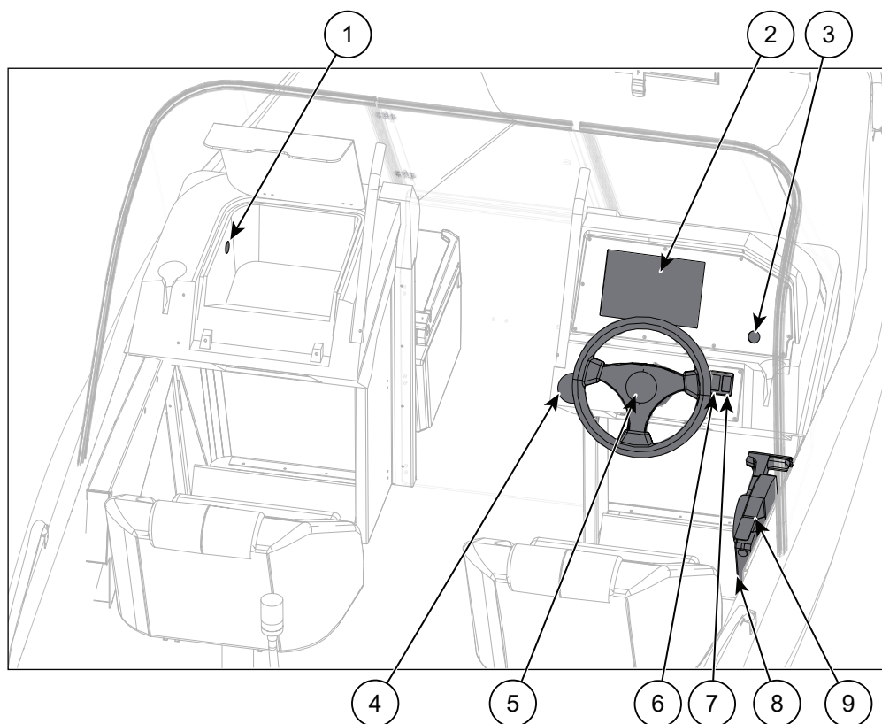
Figur 5.1 Förarplatsens kontroller på Buster X
