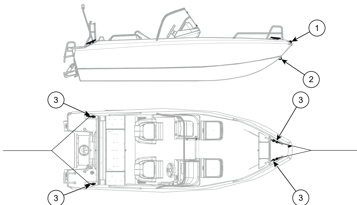
Figur 5.5 Buster X förtöjnings- och bogseringspunkter
